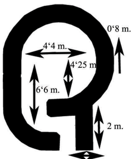
M.G.P. 001. Planta i mesures. Casamata les Deveses I.
